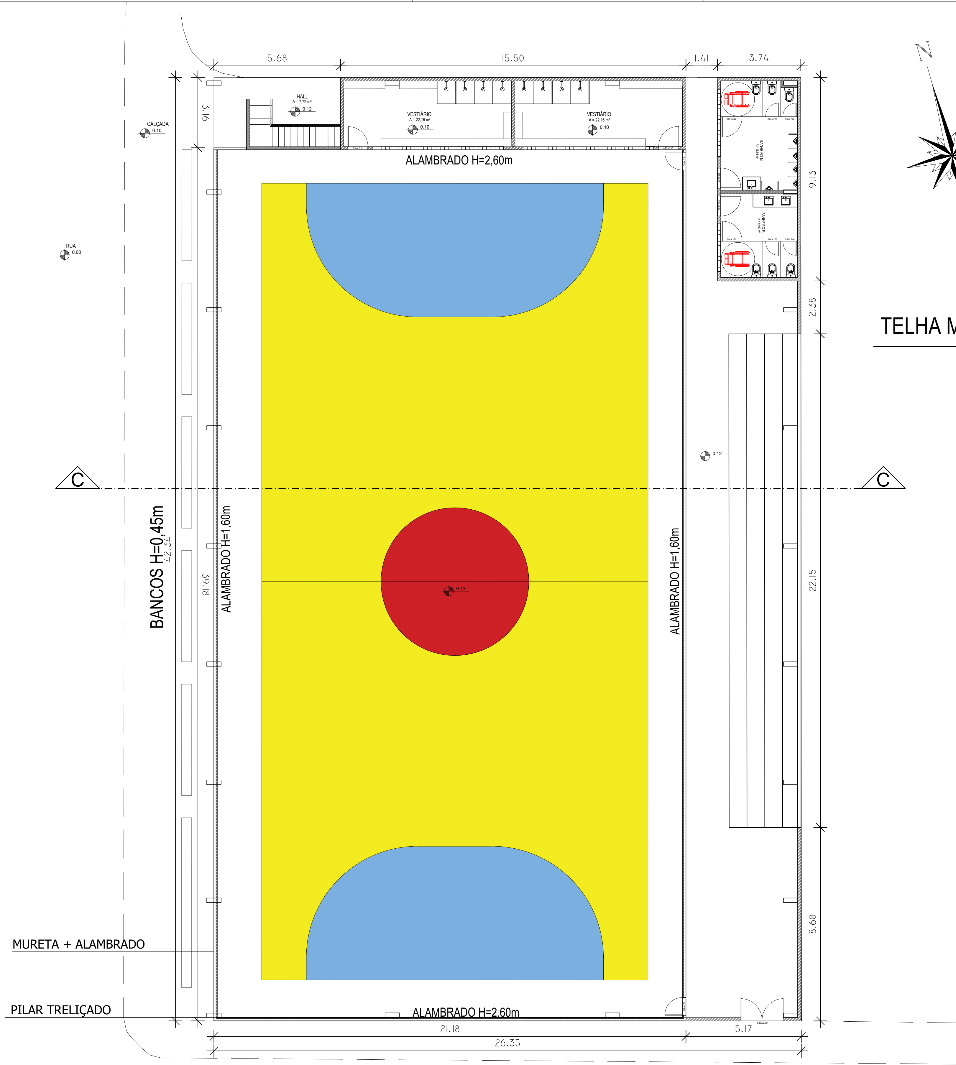
PLANTA BAIXA - QUADRA ESC. 1/100
